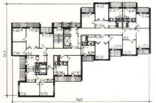
● 16-этажные жилые дома серии Т Киевпроект Архитекторы Л. Муляр, В. Таенчук Конструкторы М. Хризман, А. Иванов
