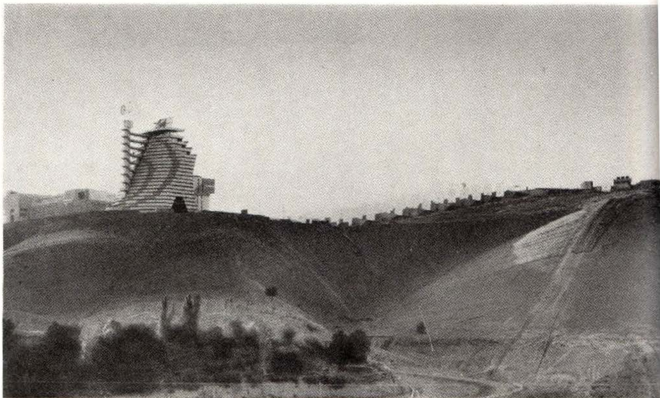
Общий вид гелиокомплекса «Солнце» из поселка Чанги
