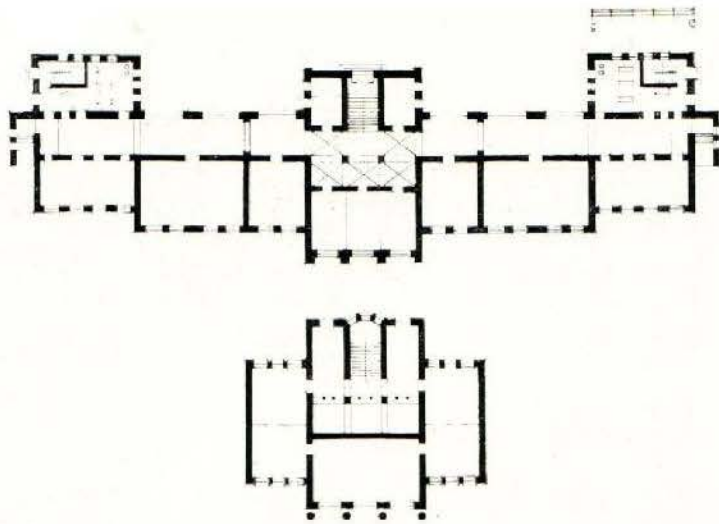
улице, 1912—1913 гг. Архитектор И. Машков Планы 1-го и 2-го этажей, общий вид
