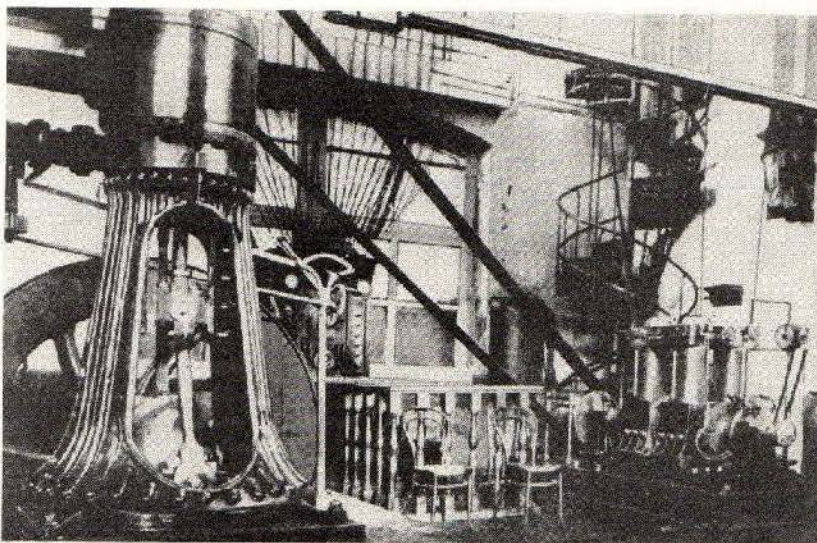
● Мартеновская фабрика Кувшинского завода. 1904 г.
