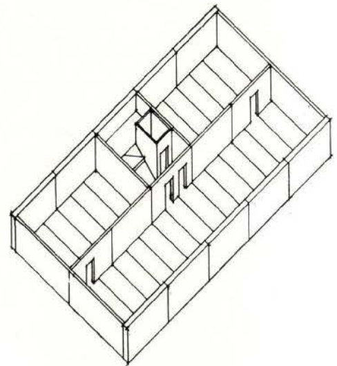
● Конструктивная схема секции с продольными несущими стенами
