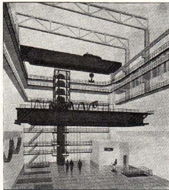
● Смоленская АЭС Блочный щит Реакторный зал
