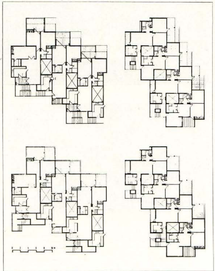
● Квартал Ямуна в Нью-Дели. 1981 г. Архитекторы Р. Сабикхи и А. Чоудхари Общий вид, планы этажей, генплан
