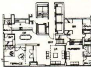
Жилой дом «Канчанджунга» в Бомбее Архитектор Ч. Корреа Общий вид, разрез, планы этажей Двухцветная лоджия
