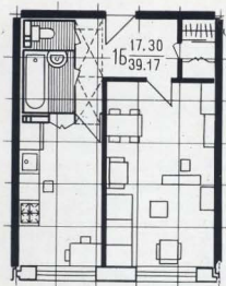
Планы однокомнатных блок-квартир
