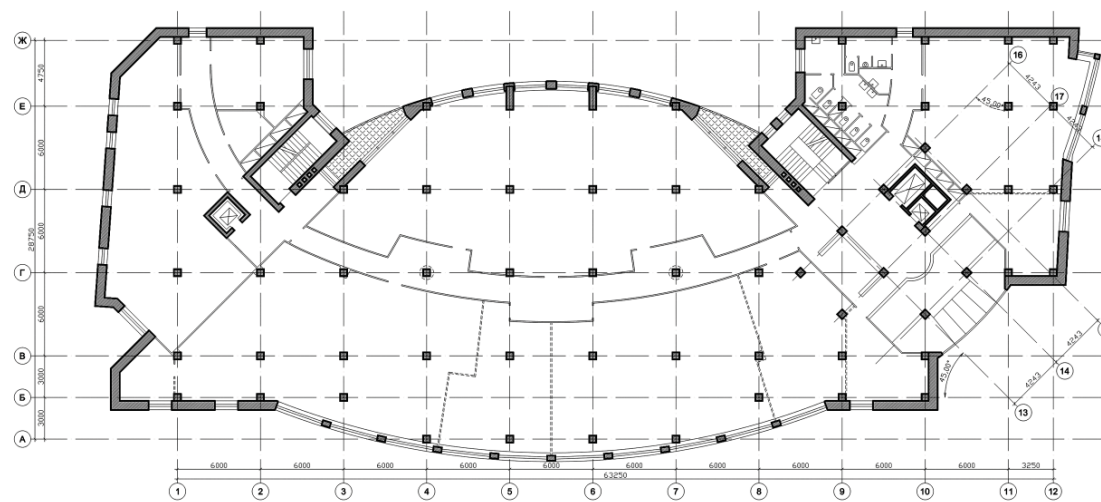
ПЛАН 2 ЭТАЖА
